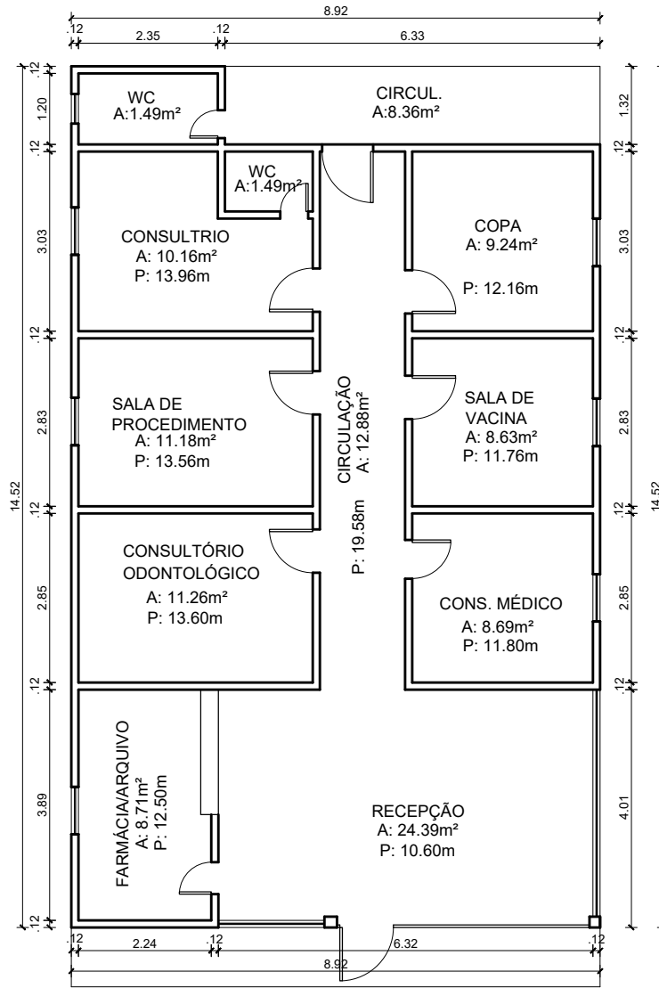
PLANTA BAIXA - ESF DE MOCAJATUBA ESC 1/100
