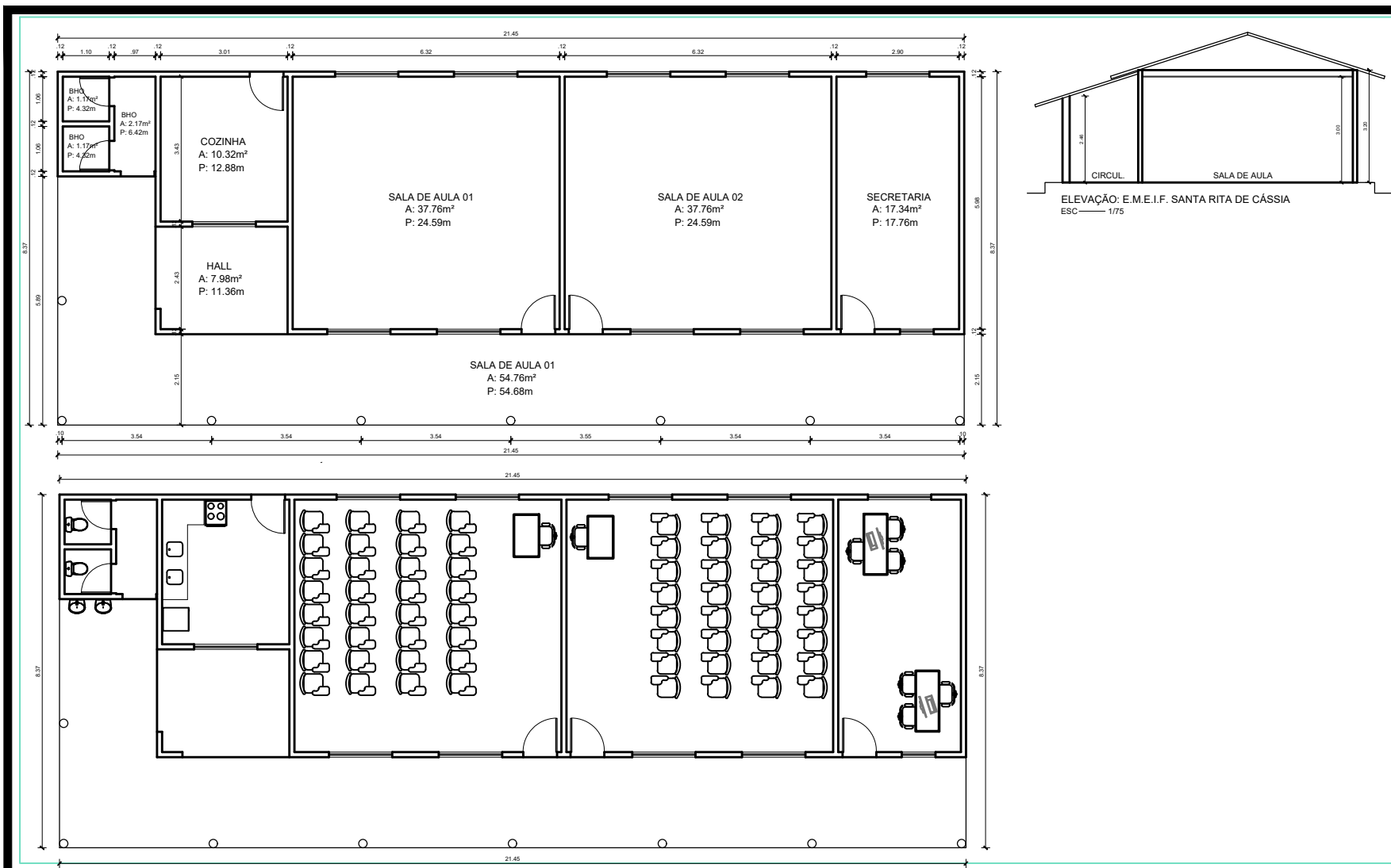
PLANTA BAIXA: E.M.E.I.F. SANTA RITA DE CÁSSIA ESC — 1/75
