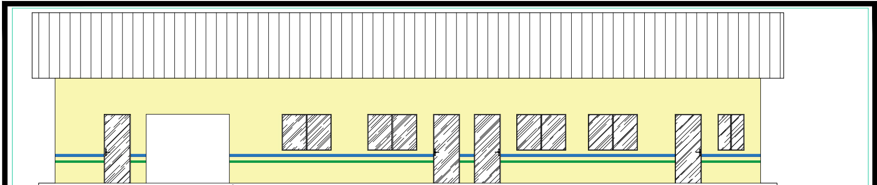
LAY OUT: E.M.E.I.F. SANTA RITA DE CÁSSIA ESC — 1/75
