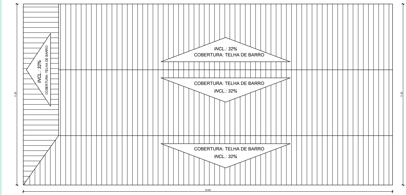
LAY OUT: E.M.E.I.F. SANTA RITA DE CÁSSIA ESC — 1/75
